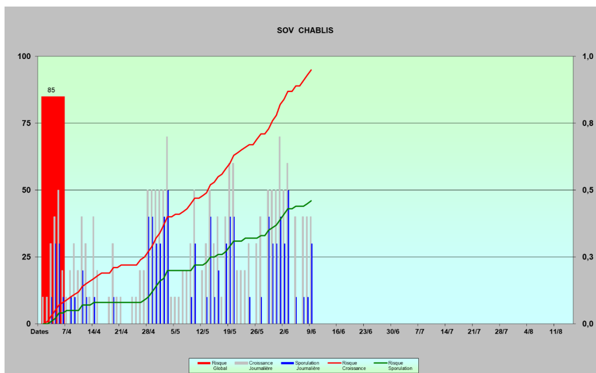
Graphique 1 : Données du modèle SOV pour le site de Chablis.
